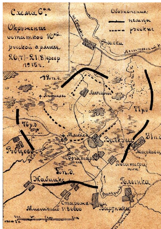
Схема окружения корпуса и 4-го СКП
